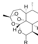
Artemisinin 1 , R = =O Artesunate 2 , R = \alpha -OC(O)CH 2 CH 2 CO 2 Na Artemether 3 , R = \beta -OMe
